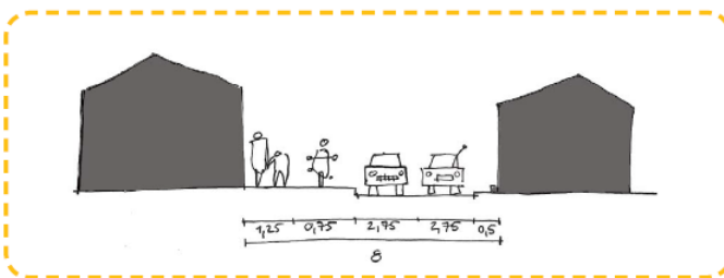
Principssnit byrum ved stationsby - smalleste sted. Mål 1:200 (alle mål i meter)
