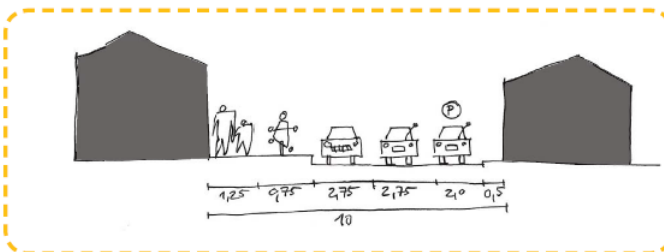
Principssnit byrum ved stationsby - bredeste sted med parkering. Mål 1:200 (alle mål i meter)
